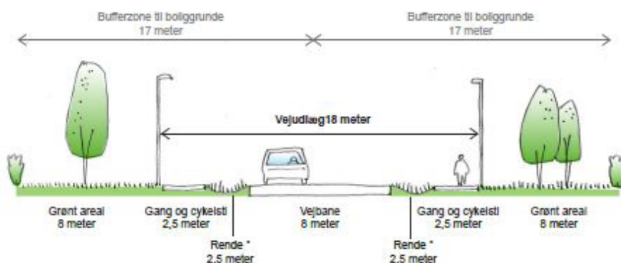
Snit i boligvej
