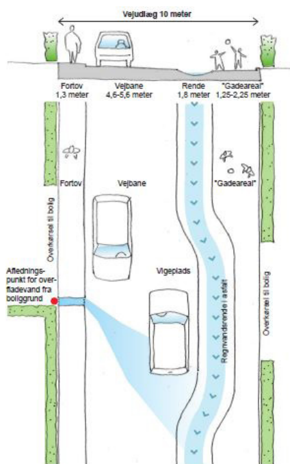
Afledning af regnvand
